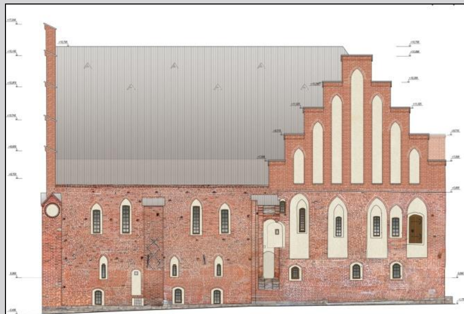
Северный фасад. Корректировка эскизного проекта реставрации. 2011 г.
